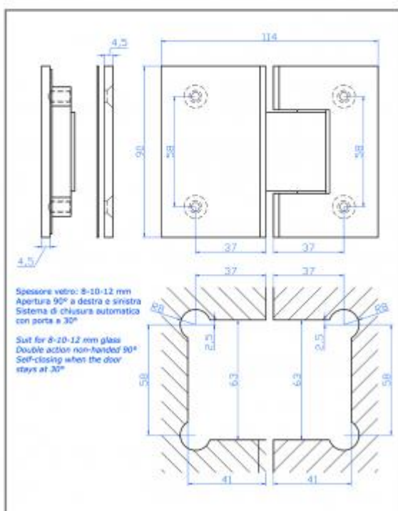
860110 cerniera vetro - vetro per box doccia
